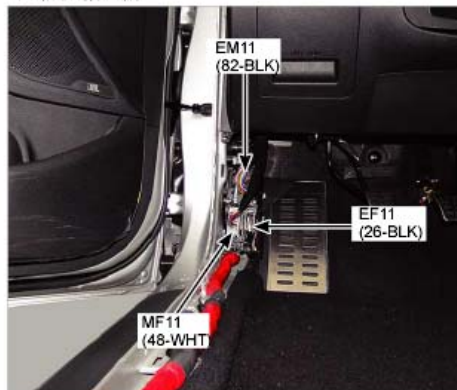
75.防火板左侧
