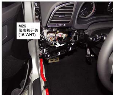
73.仪表板左侧
